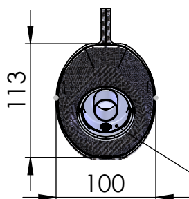
dB-Killer n°62 P/N 3014259801
